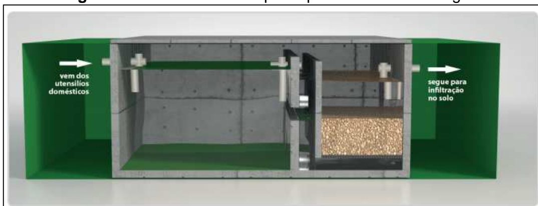
Figura 1.5 – Modelo de tanque séptico mais filtro biológico
