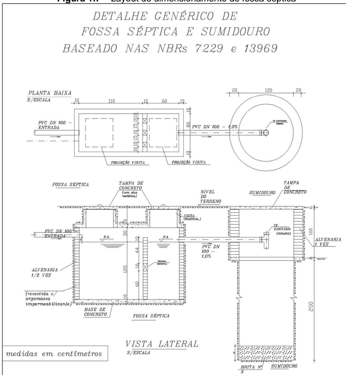
Figura 1.7 – Layout de dimensionamento de fossa séptica
