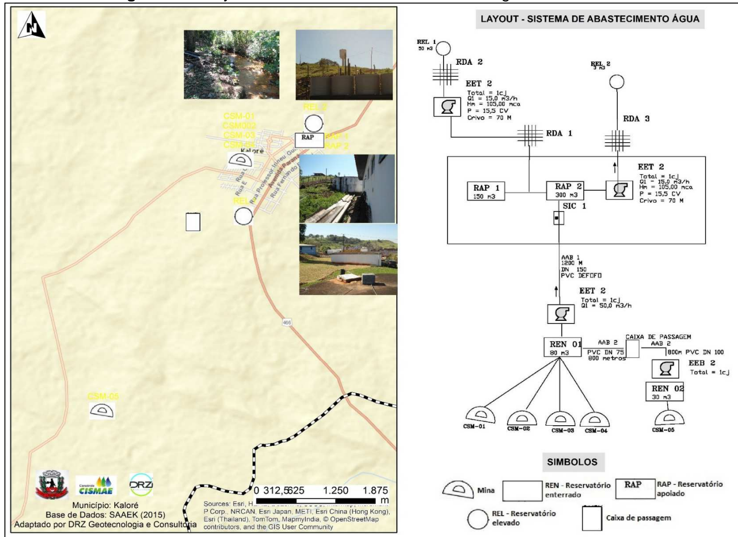
Figura 1.2 – Layout do sistema de abastecimento de água da área urbana
