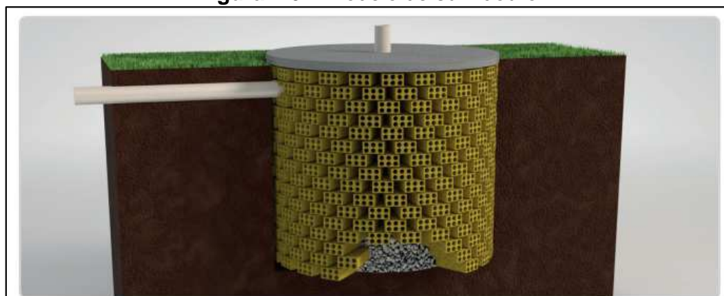
Figura 1.6 – Modelo de sumidouro
